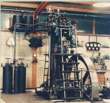
Deutz Airblast Injection 1913
